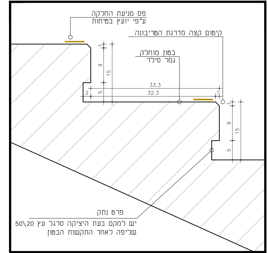
פרט P3 1:5
