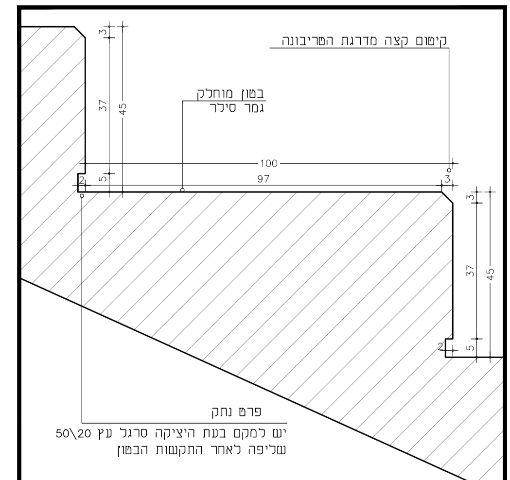
פרט P3 1:5
