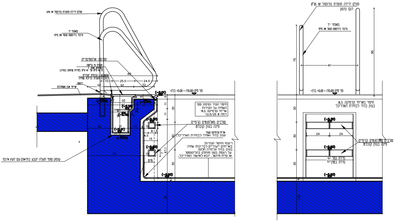
פרט ראש קיר עם סולם בריכה ראשית עומק -0.90
