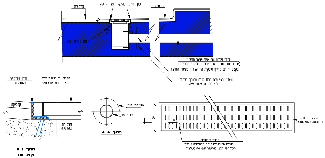
מידות: 60/400/30 פרט תעלת ניקוז בריכת פעוטות
